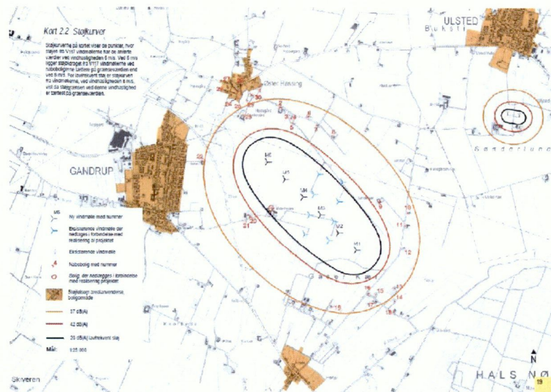
1Illustration af støjbelastning rundt om vindmøllerne. Den røde linje er beregnet til 42Db ved 6m/s og den orange linje er beregnet til 37Db, ved 6m/s.
