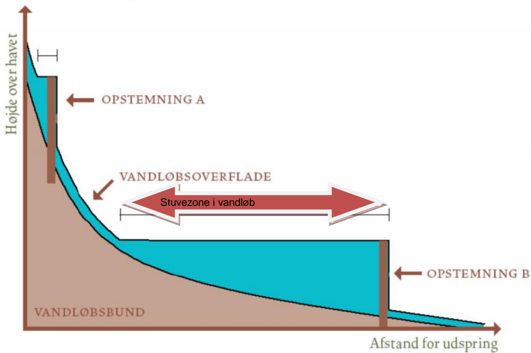
Figur 21 Illustration af stuvningszonens længde afhængig af vandløbets fald. Kilde DTU Aqua 2006, Aarestrup m.fl.
